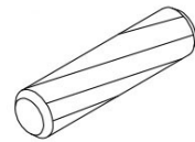
U x10 Ø8x40
